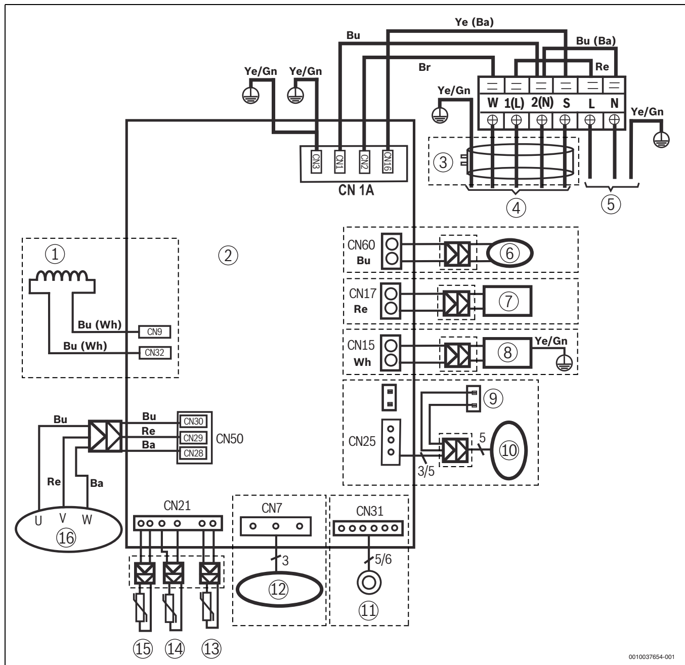
Bild 6 Schaltplan für Außeneinheiten mit 9 bis 18 kBTU/h
