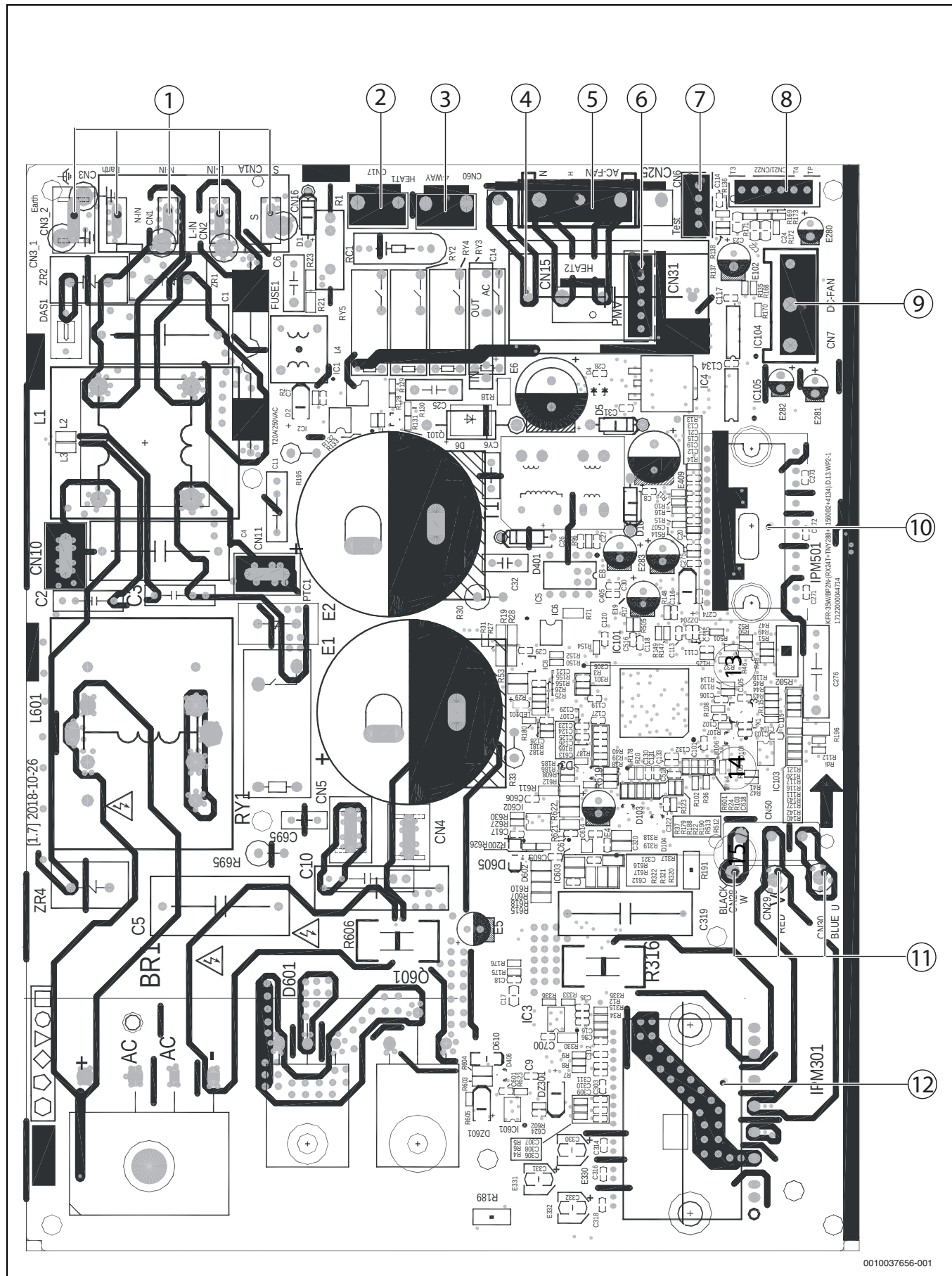
Bild 8 Hauptleiterplattenanschlüsse für Außeneinheiten mit 9 bis 18 kBTU/h
