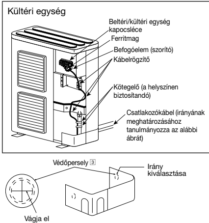
A CSATLAKOZÓKÁBEL ELVEZETÉSÉNEK RÉSZLETES ÁBRÁJA
