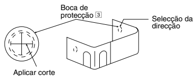
DETALHE DO GUIA DO CABO DE LIGAÇÃO
