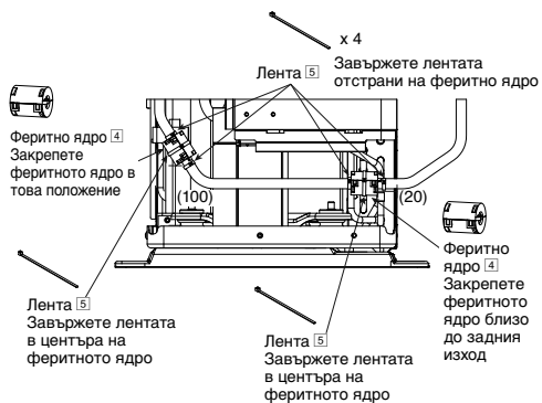
ИЗГЛЕД ОТСТРАНИ
