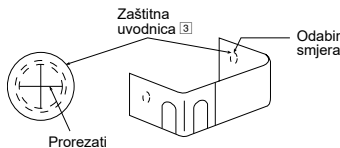
POJEDINOST POVEZIVANJA VODEĆEG KABELA
