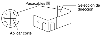
DETALLE DE LA GUÍA DEL CABLE DE CONEXIÓN
