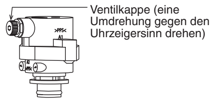
Schnellentlüfter ⑫
