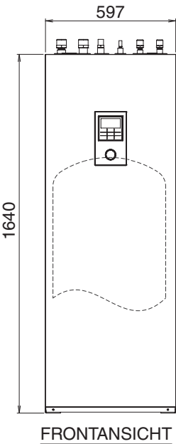
FRONTANSICHT
