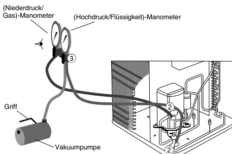
Die Beispiel-Abbildung zeigt ein Setup zur Erkennung von Kältemittel leaks.
