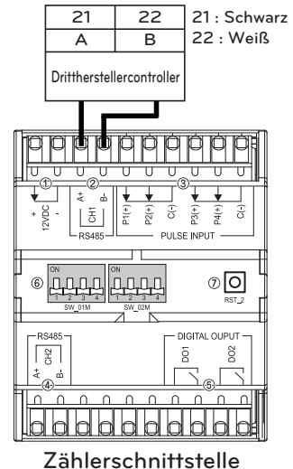
CN_MODBUS
