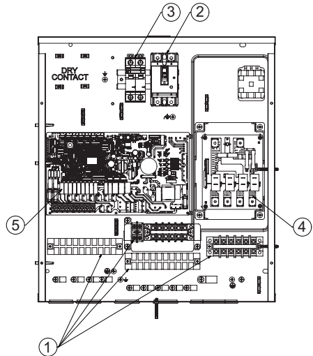
Mit Heizer-PCB
