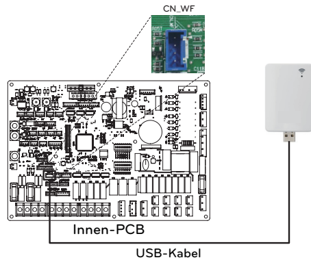
USB-Kabel
