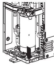
Vorgestanzte Rohrführung
