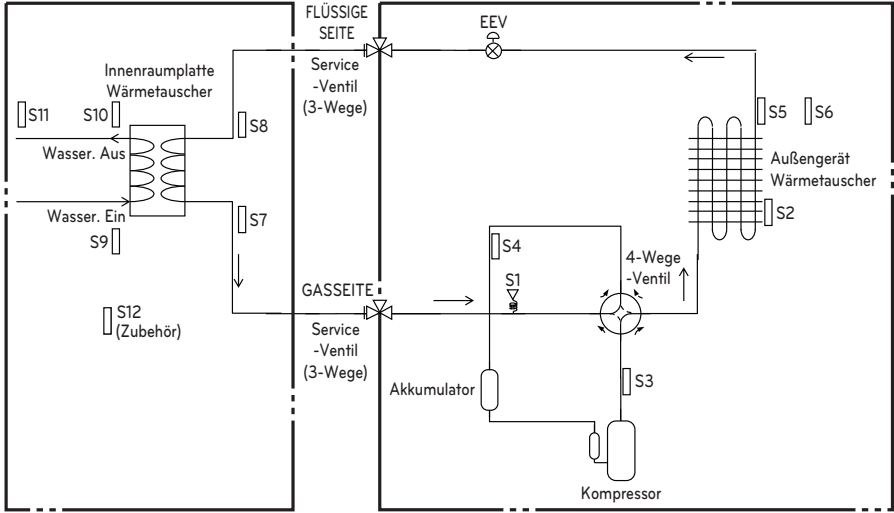
Außengerät 3 Serie
