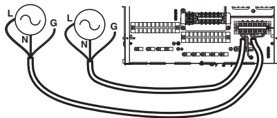
1Ø Standheizung (Für das Split-R32-Innengerät der 4er-Reihe)
