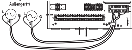
1Ø Standheizung
