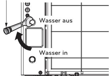
Drehmomentschlüssel
