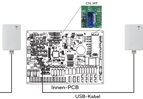
USB-Kabel
