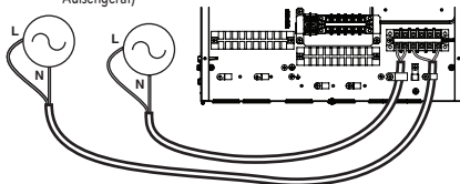
1Ø Standheizung (Für Hydrosplit)
