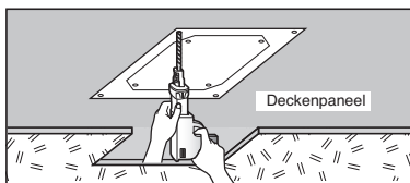
TM/TN/TP/TM-A/TP-B Gehäuse
