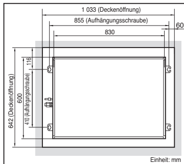
TS Gehäuse
