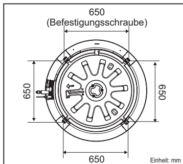
TY Gehäuse
