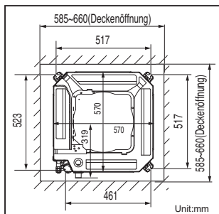
TQ/TR Gehäuse
