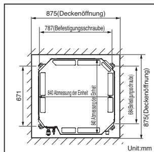
TM/TN/TP/TM-A/TP-B Gehäuse
