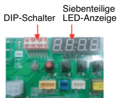
Leiterplatte des Außengerätes
