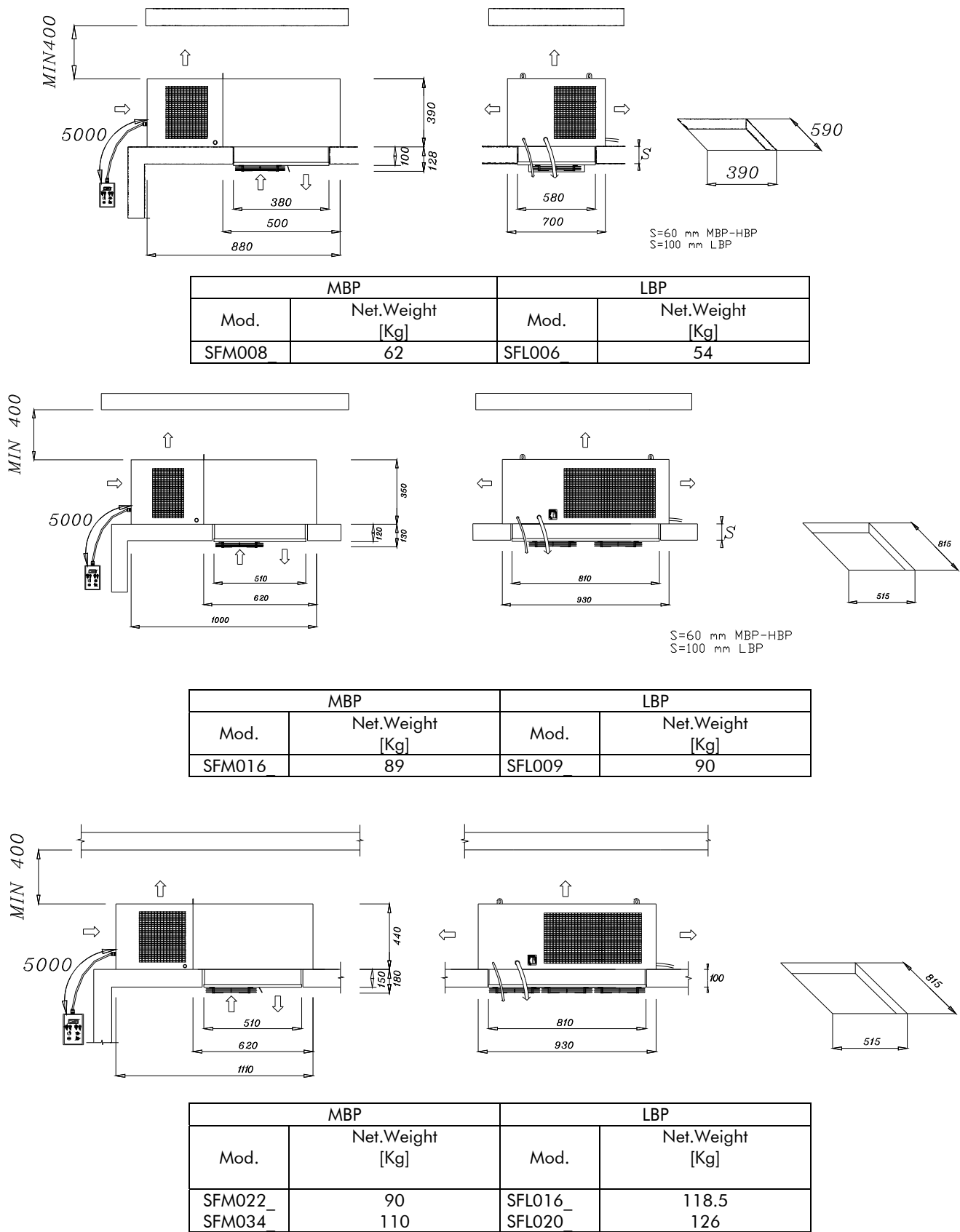
Figura 5 – Limiti dimensionali della macchina e foro da praticare sul soffitto della cella/ Macchine dimensions and hole to do on the ceiling of cooldroom
