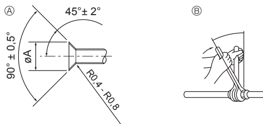
Ⓐ Abmessungen der Aufweitungsstücke Ⓑ Anzugsdrehmoment für die Konusmutter
