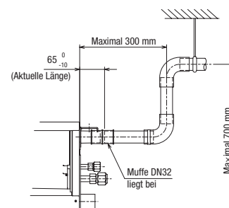
Kondensatleitungsanschlussmaße
