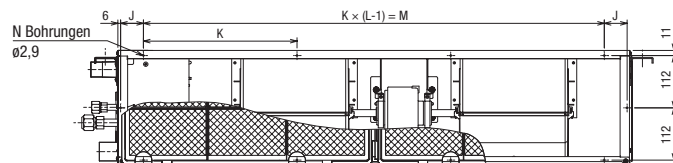
Rückluftkanalanschlussmaße (Eintritt)
