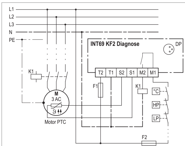
Anschluss-Schaltbild
