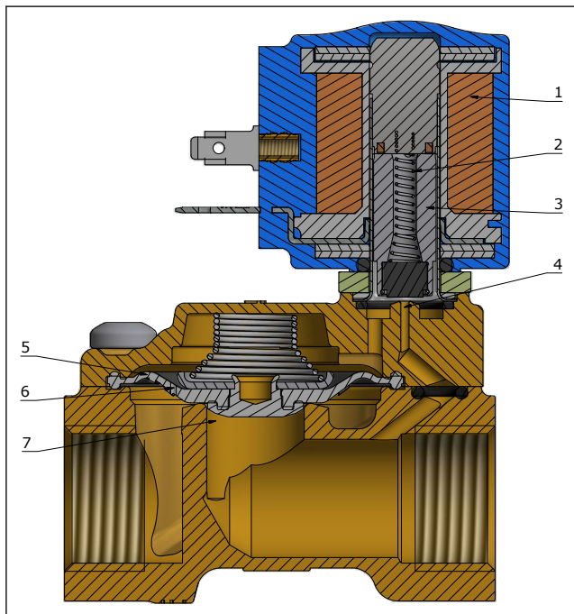
Bild 1: Funktion, NC
