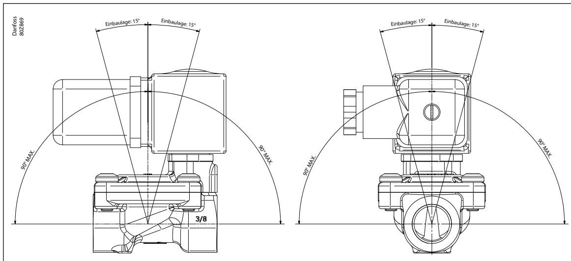
Bild 7: Montagewinkel
