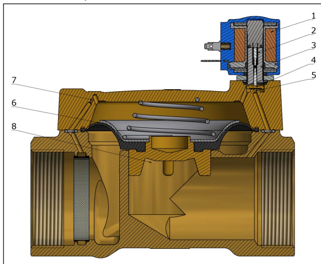
Bild 2: Funktion, NO
