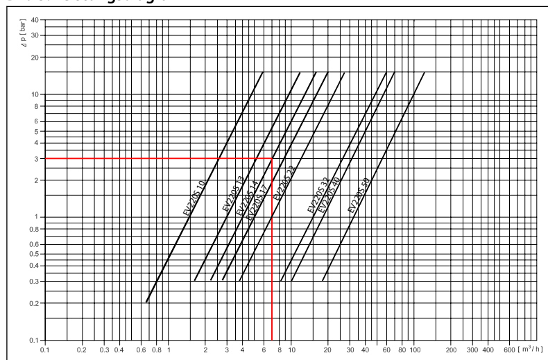
Bild 5: Leistungsdiagramm
