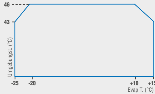
MODELL SIL AJV 9513 Z SIL AGV 4553 Z
