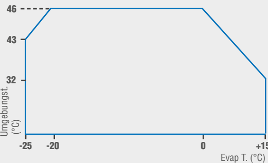
MODELL SIL FHV 4540 Z
