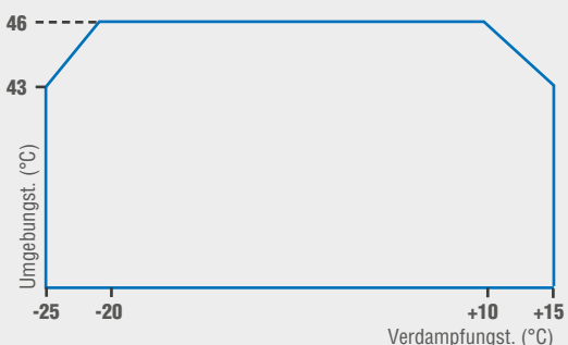
MODELL SIL AJV 4492 Y SIL AGV 4543 Y
