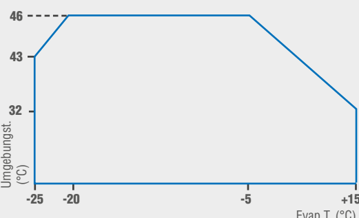
MODELL SIL SHV 4610 Z
