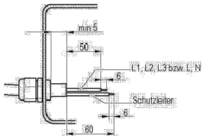
Abb. 1: Empfohlene Abmantellungslängen in mm (innerhalb Klemmkasten)
